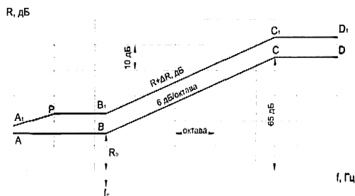
Рисунок 6 - Построение частотной характеристики изоляции воздушного шума стеной с гибкой плитой на относительное
