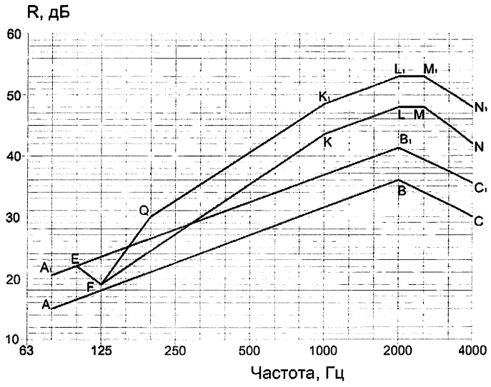
Рисунок А.3 - Расчетная частотная характеристика
