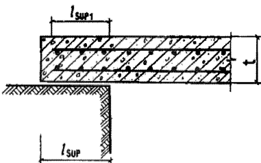
Рисунок 7.1 – Схема свободного опирания плоских изгибаемых элементов
