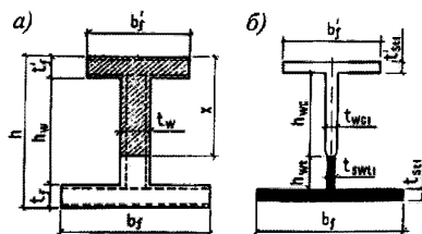
Рисунок 6.14 – Схема приведения сечения армоцементных элементов к стальному
