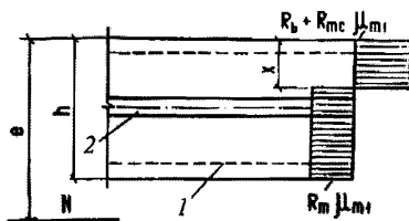
Рисунок 6.12 – Эпюра напряжений во внецентренно растянутых элементах прямоугольного сечения при приложении продольной силы N за пределами сечения
