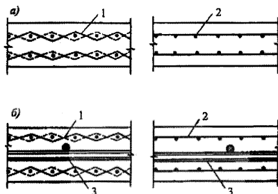
Рисунок 4.1 – Армирование армоцементных конструкций
