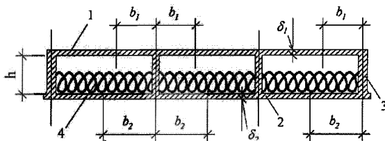
Рисунок 6.1 – Поперечное сечение каркасной плиты
