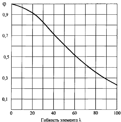
Рисунок 6.9 – График для определения коэффициента продольного изгиба φ
