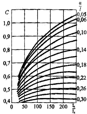
Рисунок 6.5 – График для определения коэффициента C
