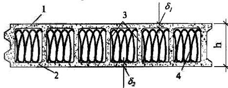
1, 2 – полки панели; 3 – ребра панели; 4 – утеплитель.
