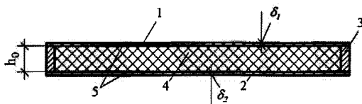
Рисунок 6.4 – Поперечное сечение бескаркасной панели с обрамлением
