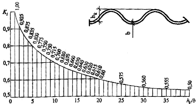
Рисунок 6.6 – График для определения коэффициента K_1
