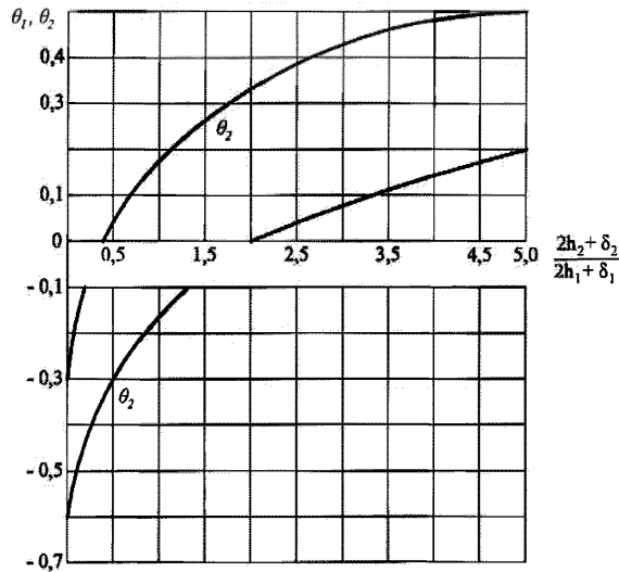
Рисунок 6.7 – График для определения коэффициентов \theta_1 и \theta_2
