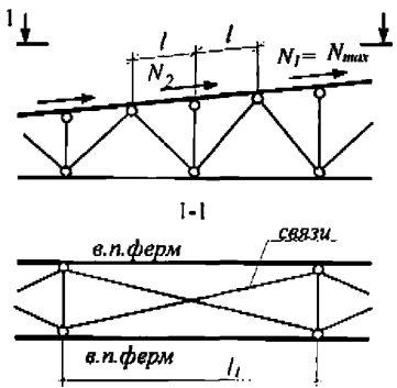
Рисунок 9 – Схемы для определения расчетной длины элементов
