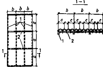
1 – продольные ребра; 2 – поперечные ребра
