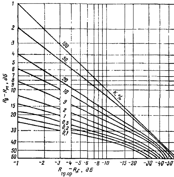
Рисунок 15 – Номограмма для определения средней звукоизоляции неоднородных ограждений
