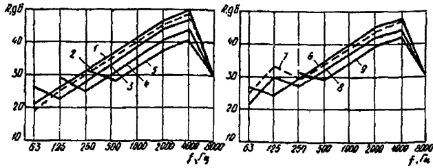
Рисунок 4 – Звукоизоляция пластины из стали толщиной от 1,5 до 2,0 мм разных размеров
