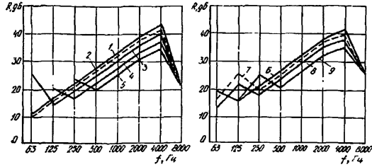
Рисунок 10 – Звукоизоляция пластин из органического стекла толщиной от 3 мм до 4 мм разных размеров
