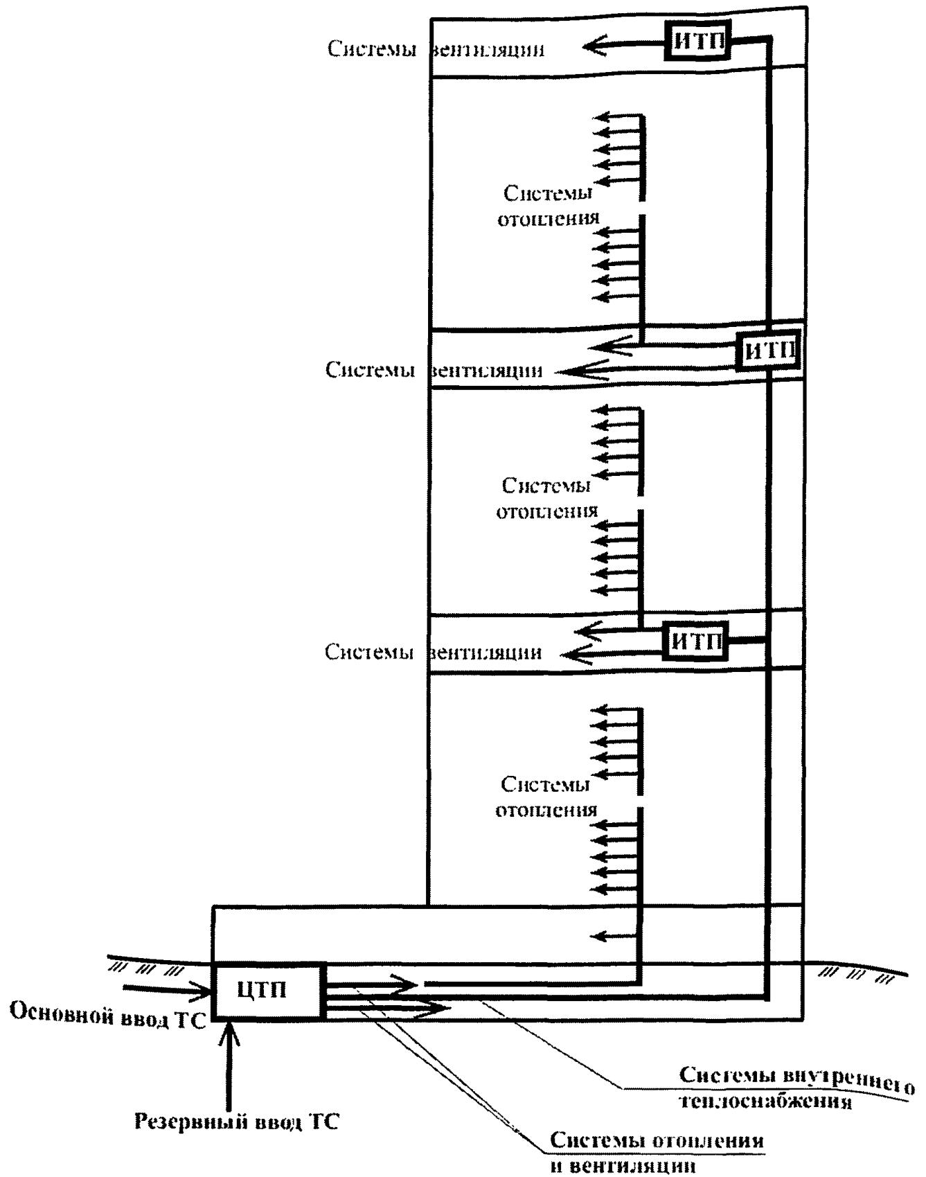
Рисунок 5.1 – Схема теплоснабжения высотного здания от централизованного источника
