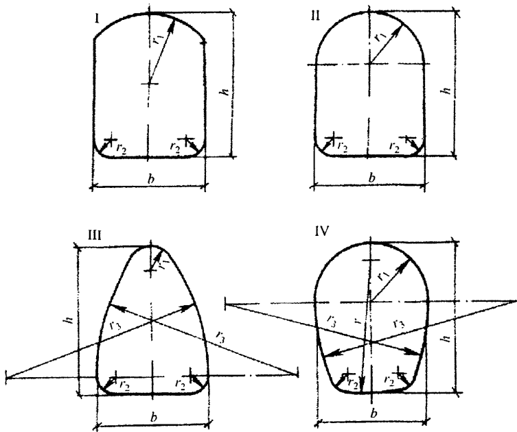
Рисунок 1 – Формы поперечных сечений безнапорных туннелей в свету
