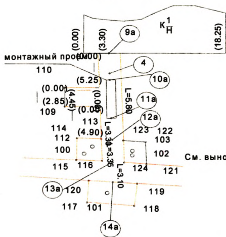
СХЕМА ПРОМЕРОВ
