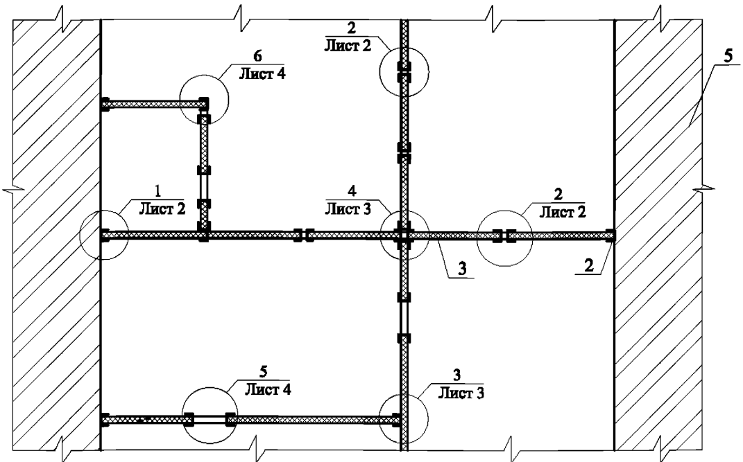
ориентация покровных слоев панели при монтаже
