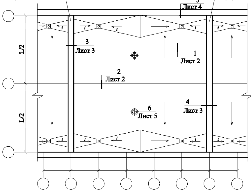
деформационный шов (продолжение) противопожарный пояс
