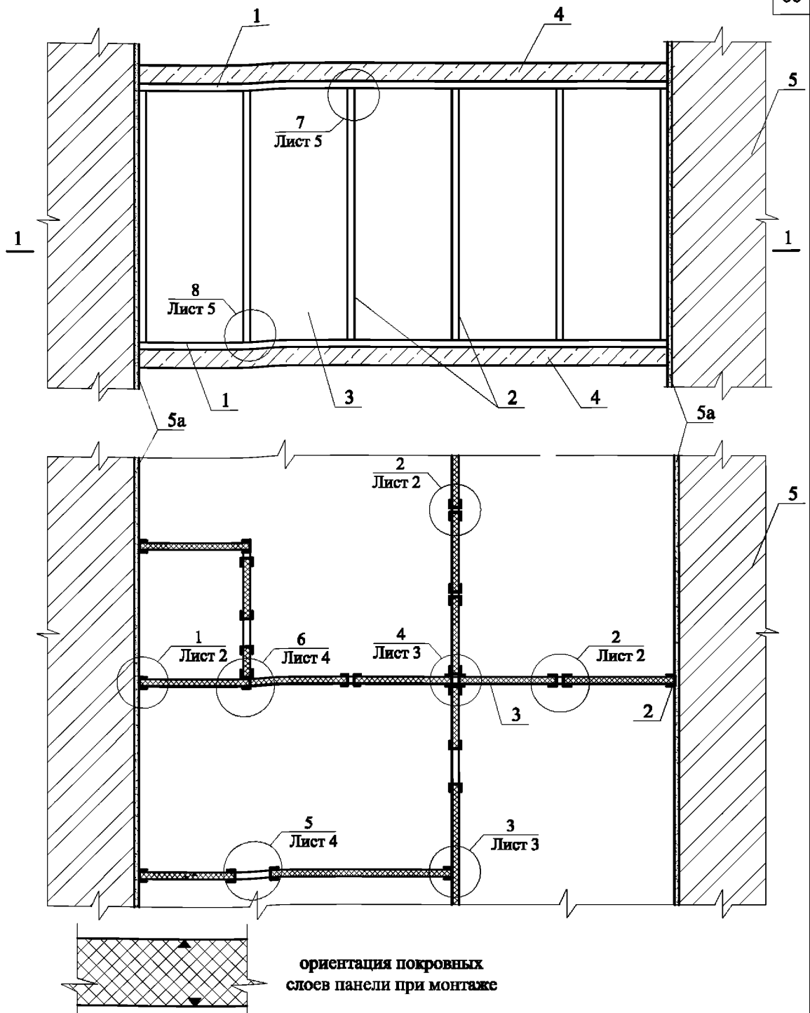
1-деревянный брус 50хбпан (бпан-толщина панели БАРЛАЙТ); 2- стойка каркаса; 3-панели БАРЛАЙТ; 4-междуэтажное перекрытие; 5-стена; 5а - внутренний отделочный слой стены.
