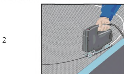
Рисунок 11.1. Забивка труб (канализации, отопления и т.п.) панелями БАРЛАЙТ 1 – общий вид короба (поперечный разрез); 2 – разделка внутреннего угла панели строительным ножом или фрезой; 3 – склейка короба монтажной пеной; 4 – крепления короба к стенам.
