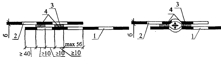
Рис 5. Испытание сварного шва с испытательным каналом
