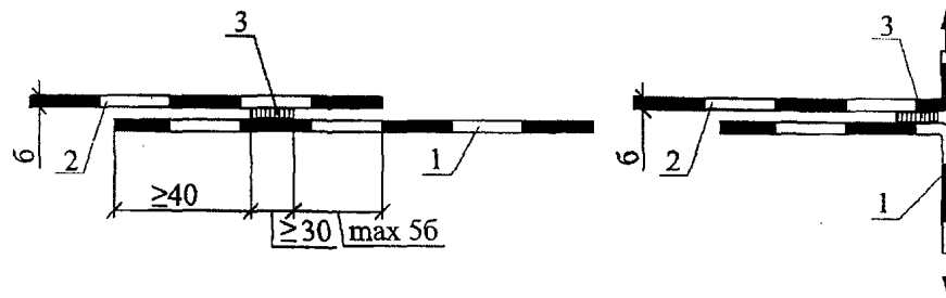
Рис.4. Испытание сварного шва внахлестку
