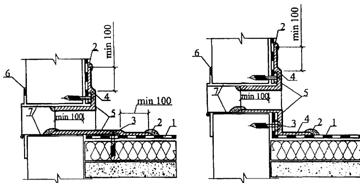
Рис.1. Водоотвод с кровли через парапет (стену)
