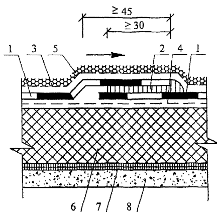
Рис. 2 Свободная укладка (балластная система) мембраны «ЮНИФОЛ»
