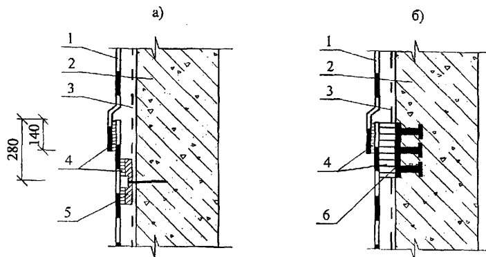
Рис. 6 Крепление полотнищ мембраны «ЮНИФОЛ» к стене при помощи планки (а) и закладной детали (б)
