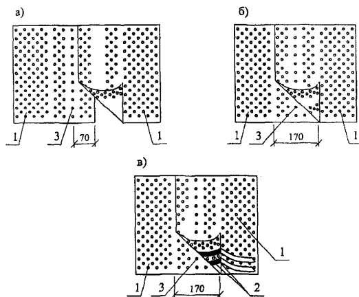
Рис. 7. Стык продольных кромок мембраны «ЮНОП»
