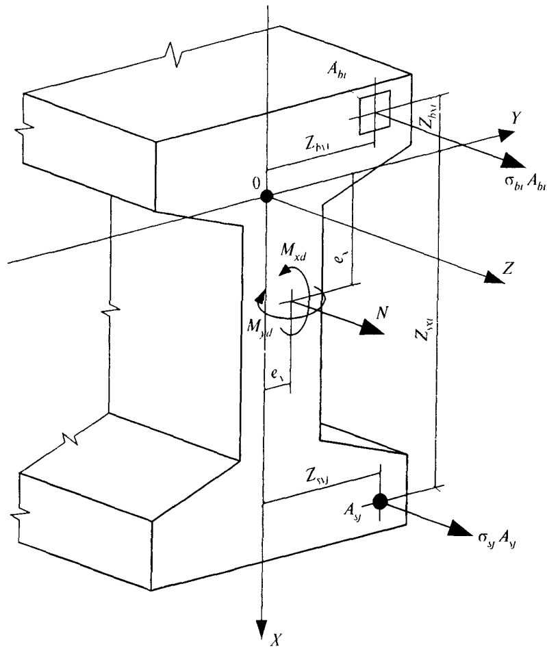
Рисунок 6 — Расчетная схема нормального сечения железобетонного элемента
