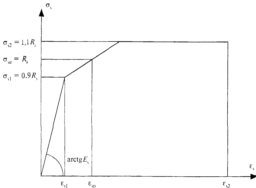
Рисунок 2 — Диаграммы состояния растянутой арматуры
