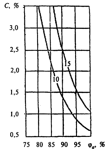
Рисунок Ш.2 — Изолинии сорбционного влагосодержания керамзитобетона \rho_0 = 1200 \text{ кг/м}^3 , содержащего хлорид калия, при изменении относительной влажности воздуха \varphi_v, \% , и массового солесодержания C, \%
