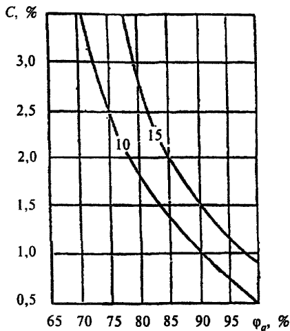
Рисунок Ш.1 — Изолинии сорбционного влагосодержания керамзитобетона \rho_0 = 1200 \text{ кг/м}^3 , содержащего хлорид натрия, при изменении относительной влажности воздуха \varphi_v, \% , и массового солесодержания C, \%
