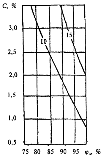
Рисунок Ш.3 — Изолинии сорбционного влагосодержания керамзитобетона \rho_0 = 1200 \text{ кг/м}^3 , содержащего хлорид магния, при изменении относительной влажности воздуха \varphi_v, \% , и массового солесодержания C, \%
