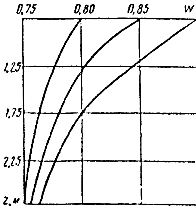
Рис.П.2.1 Номограмма для определения относительной влажности W от толщины Z_1 стабильного слоя.
