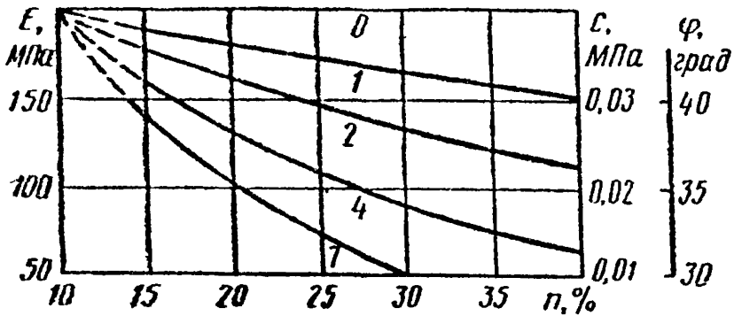
Рис П 3 1 Зависимость модуля упругости E от содержания частиц n размером менее 0,63 мм (или показателя дробимости малопрочного щебня) для щебеночных и гравийных материалов (смесей). На кривых показано число пластичности частиц в смеси размером мельче 0,63 мм.
