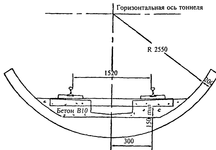
Перегонный тоннель с железобетонной обделкой
