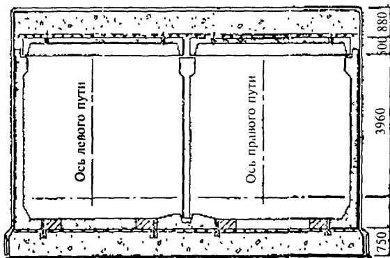
Рис. Г.1 — Конструкции тоннельных обделок
