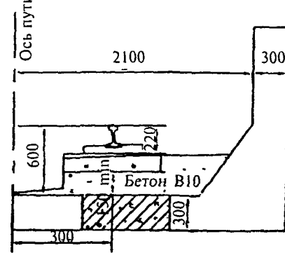
Станция мелкого заложения
