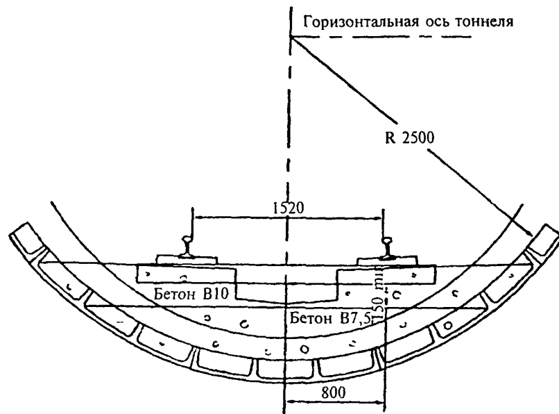
Перегонный тоннель с чугунной обделкой
