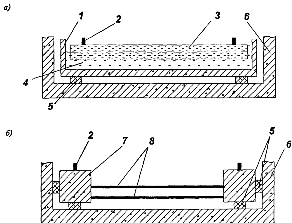
а — амортизаторами под конструкцией верхнего строения пути; б — амортизаторами под лежнями 1 — балластное корыто; 2 — рельс; 3 — шпала; 4 — щебеночная постель; 5 — амортизатор; 6 — обделка тоннеля; 7 — лежень; 8 — стальные связи
