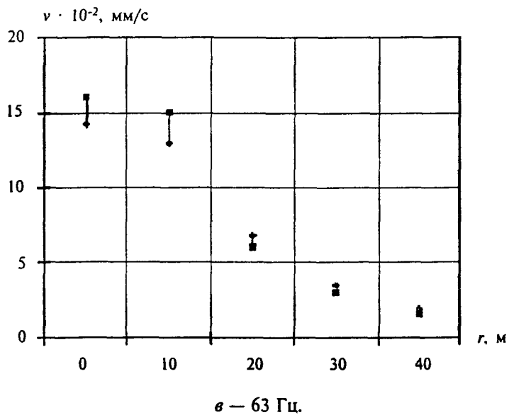
Рисунок Е.1 — Измеренные и рассчитанные значения виброскорости
