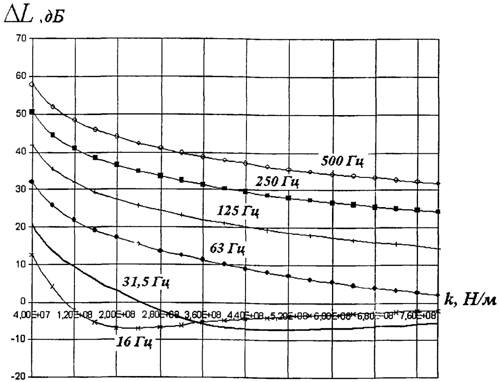
Рисунок 5.9 — Зависимость эффективности виброзащитной конструкции (вариант 2) от жесткости амортизаторов, приведенной к длине вагона, для случая грунтов со скоростью продольных волн 600 — 1200 м/с
