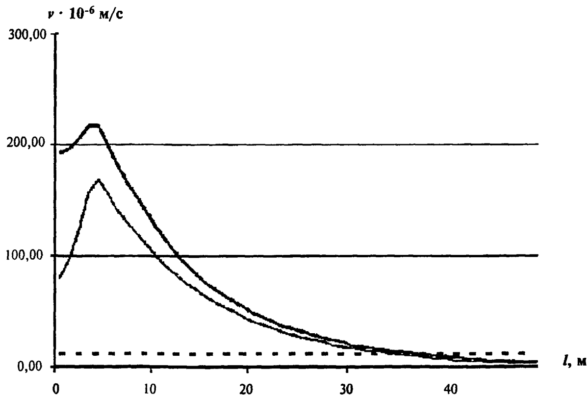
Рисунок Б.2 — Зависимость максимальной величины вертикальной и горизонтальной составляющих виброскорости v от расстояния до тоннеля l в октавном диапазоне 31,5 Гц
