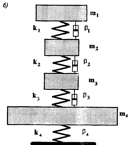
а — механическая схема; б — физическая модель системы
