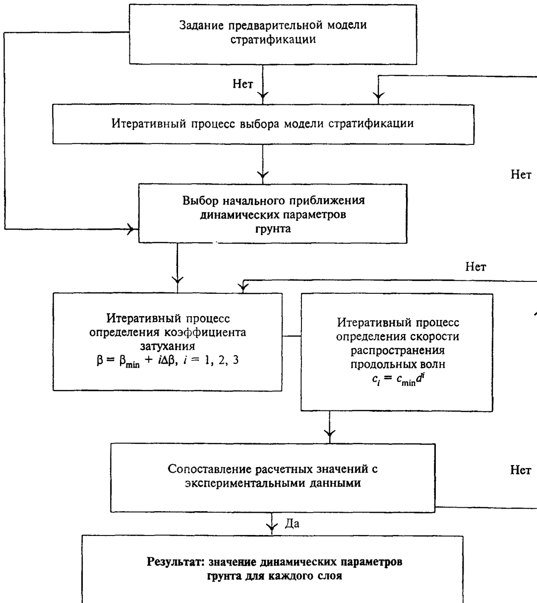
Рисунок 4.1 — Блок-схема реализации алгоритма определения динамических параметров грунта. «Да» и «Нет» означают соответственно выполнение и невыполнение условий совпадения расчетных и измеренных данных
