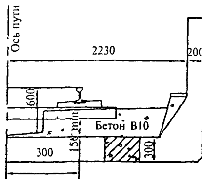
Перегонный тоннель прямоугольного сечения из железобетонных блоков
