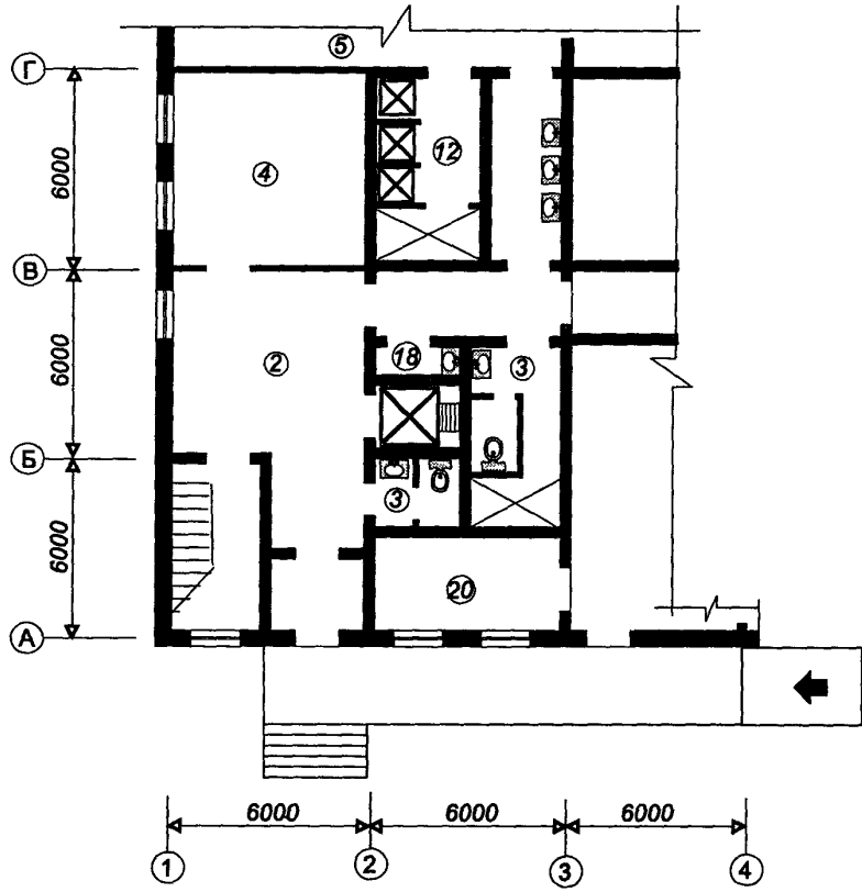
Фрагмент плана на отм. 0.000
