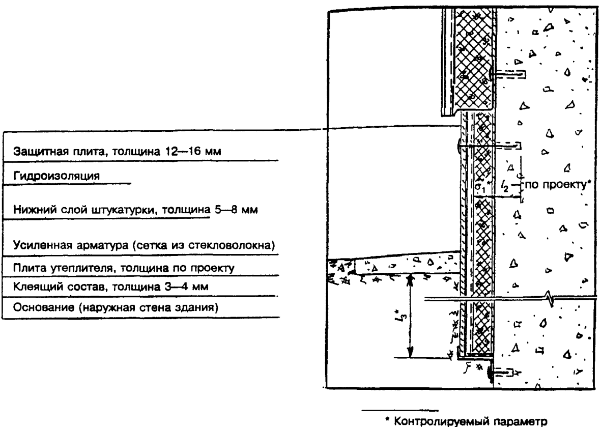
Рисунок А10 — Фрагмент утепления нижней (и ее заглубленной) части стены здания
