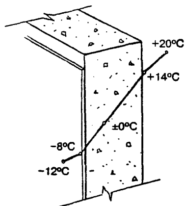
Рисунок 1 — Температурная кривая зимой
