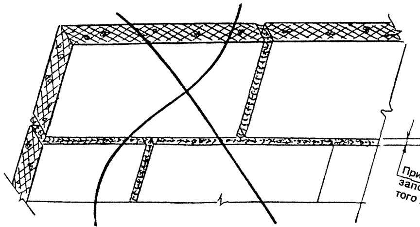
Рисунок А2 — Наклейка плит утеплителя на поверхность стены способом «перевязки»
