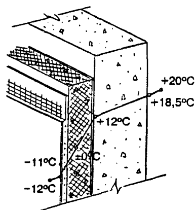
б) Наружная стена с теплоизоляцией толщиной 75 мм
