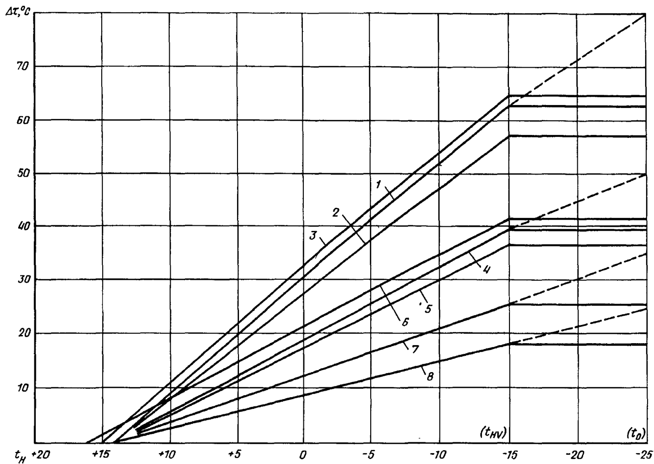
Рис. 6. Графики изменения разности температуры воды в подающем и обратном трубопроводах системы отопления \Delta t в зависимости от t_{\text{н}}
