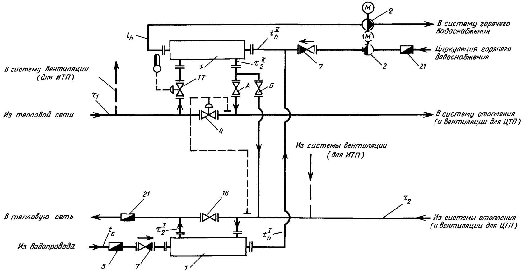
Рис. 8. Двухступенчатая схема присоединения водоподогревателей горячего водоснабжения с зависимым присоединением систем отопления при отсутствии регуляторов расхода тепла на отопление в ЦТП и ИТП
