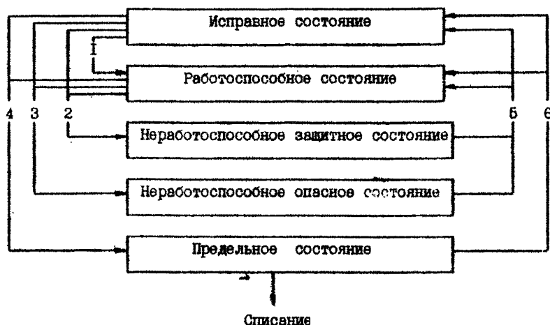
Рис.3. Схема основных состояний и событий: 1 - повреждение; 2 - защитный отказ; 3 - опасный отказ; 4 - переход системы в предельное состояние из-за неустраняемого нарушения требований безопасности, снижения эффективности эксплуатации, морального старения и других факторов; 5 - восстановление; 6 - ремонт
