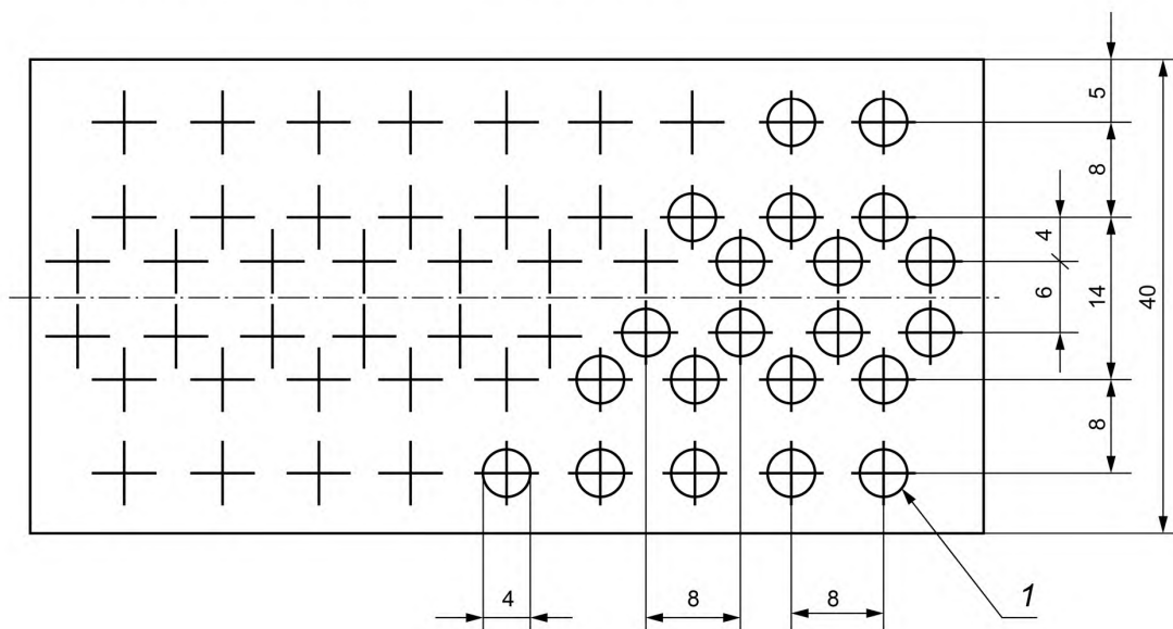
Рисунок А.1 — Конструкция щетки
