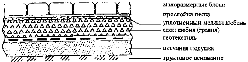
Рисунок 6 – Блочные покрытия
