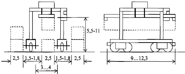
Рисунок 3 – Портальный автопогрузчик
