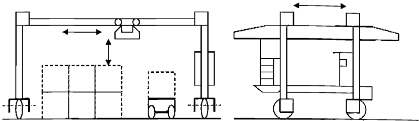
Рисунок 5 – Мостовой порталный контейнерный кран на пневмоходу
