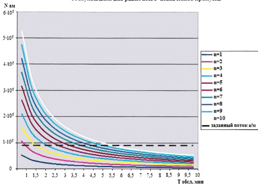
Рисунок Б.1 – Пропускная способность АВК
