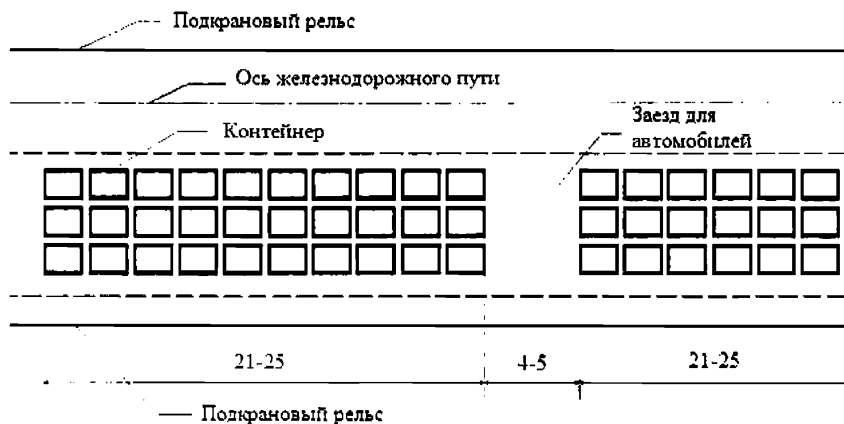
Рисунок 4 – Схема поперечного заезда автомобилей
