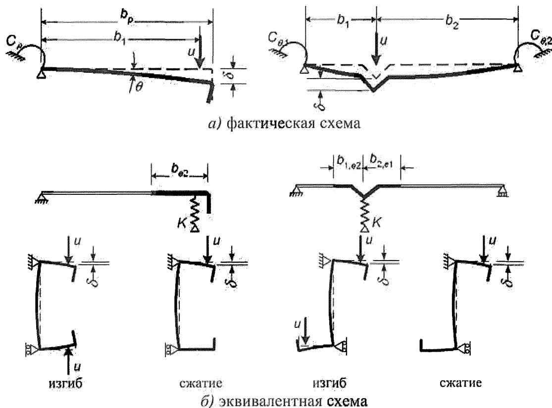
Рисунок 7.7 – Схемы к определению жесткости связей
