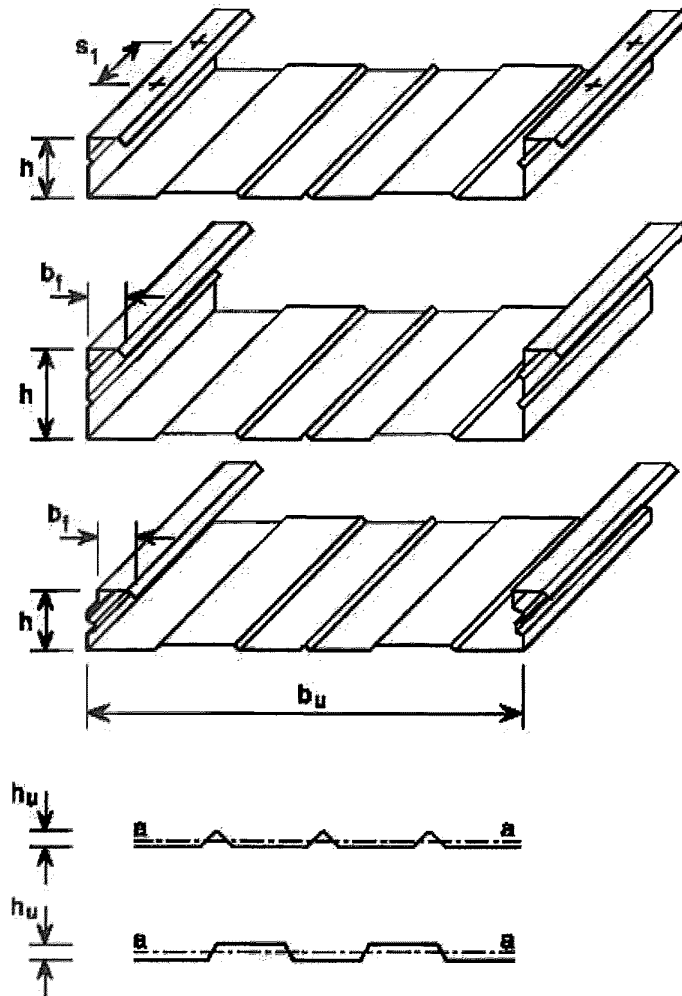
Рисунок 8.1 – Типовая геометрия кассетных профилей
