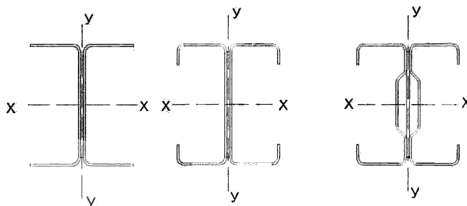
Рисунок 7.19 – Сечения сплошных стержней колонн и стоек
