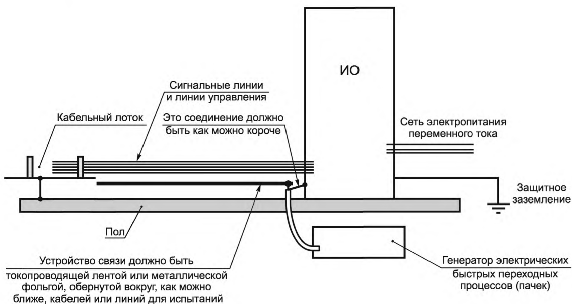
Рисунок 16 — Пример испытаний на месте установки на сигнальных портах и портах управления без емкостных клеммной связи
