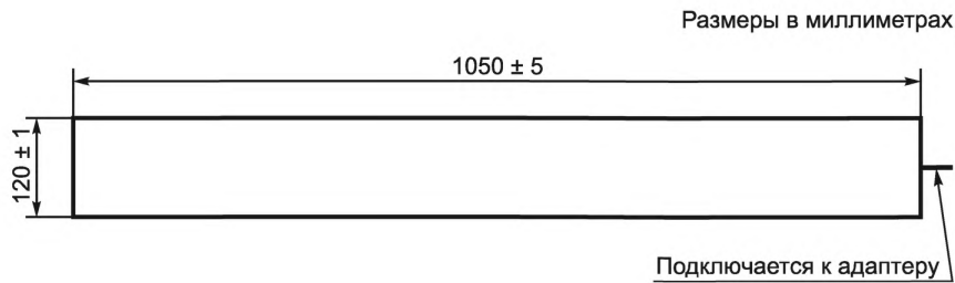
Рисунок 7 — Преобразовательная пластина для калибровки клещей связи
