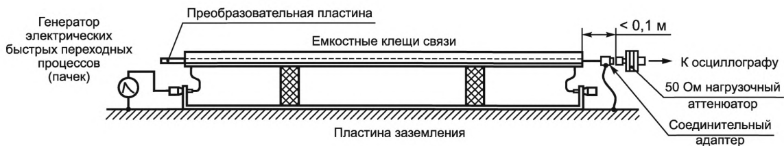
Рисунок 8 — Калибровка емкостных клещей связи с использованием преобразовательной пластины
