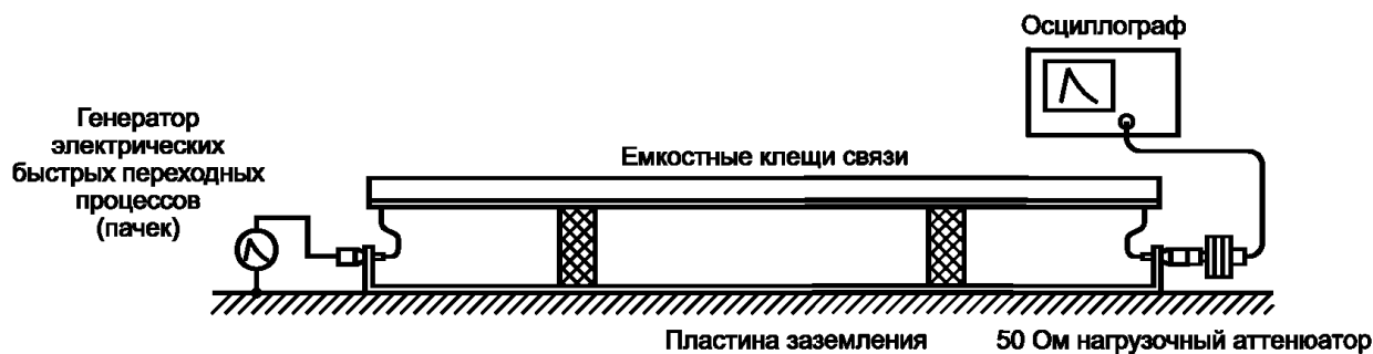
Рисунок 10 — Пример проверки емкостных клещей связи
