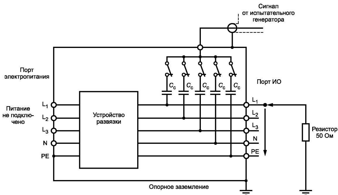
Рисунок 5 — Калибровка формы сигнала на выходе устройства связи/развязки
