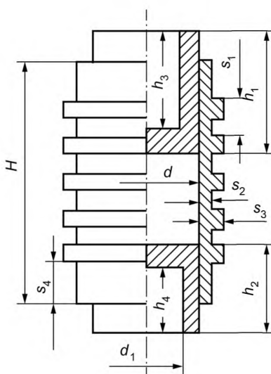
Рисунок Л.2 — Облегченная форма для уплотнения смесей
