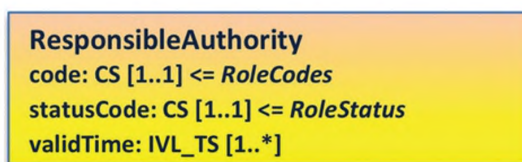
Рисунок 5 — Класс ResponsibleAuthority
