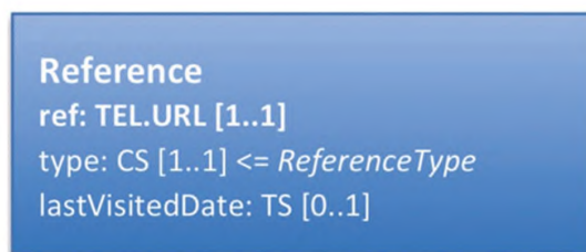
Рисунок 8 — Класс Reference
