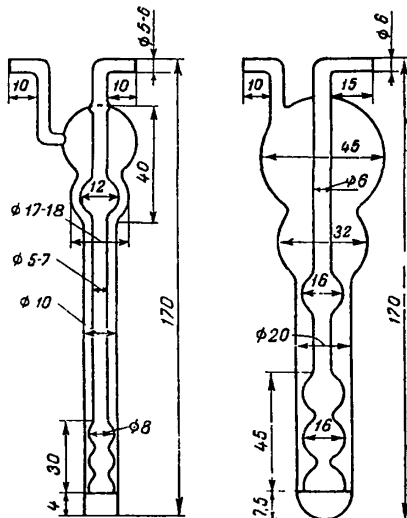
Рис. 10. Поглощительные приборы Рыхтера
