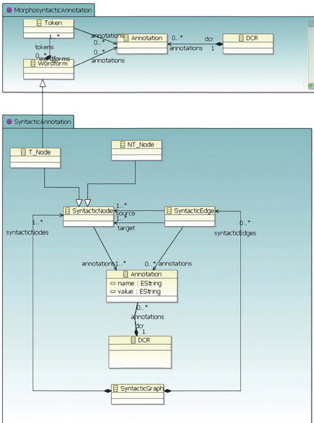
Рисунок 1 — Метамодель SynAF (скомпонованная средствами MAF)
