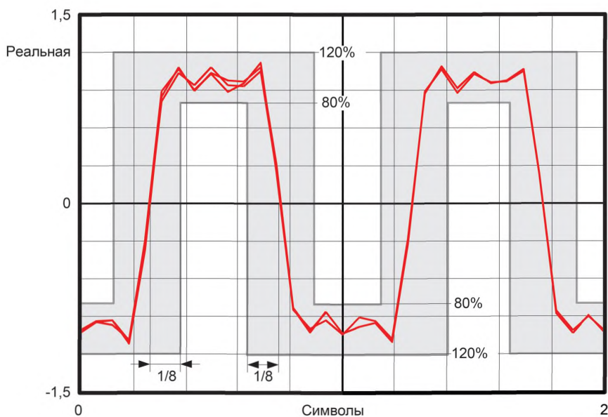
Рисунок 4 — Индикаторная диаграмма и границы измерений для BPSK модуляции
