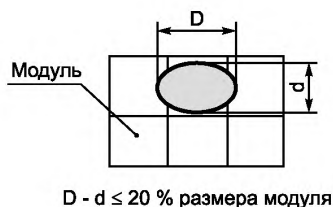
Рисунок 5 — Определение овальности
