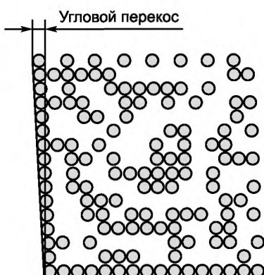
Рисунок Е.2 — Угловой перекося символа
