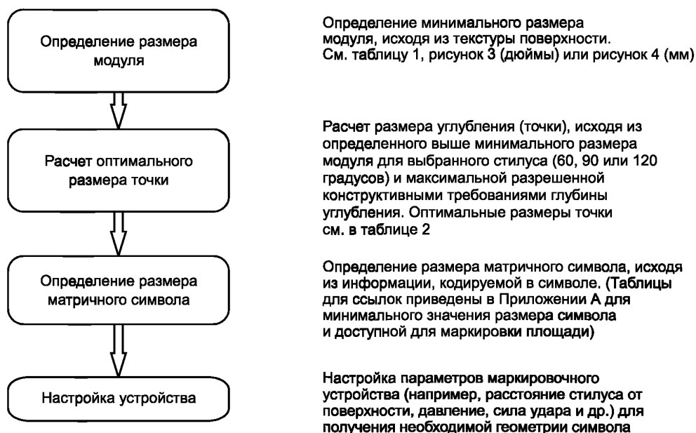
Рисунок 2 — Последовательность определения параметров маркирования
