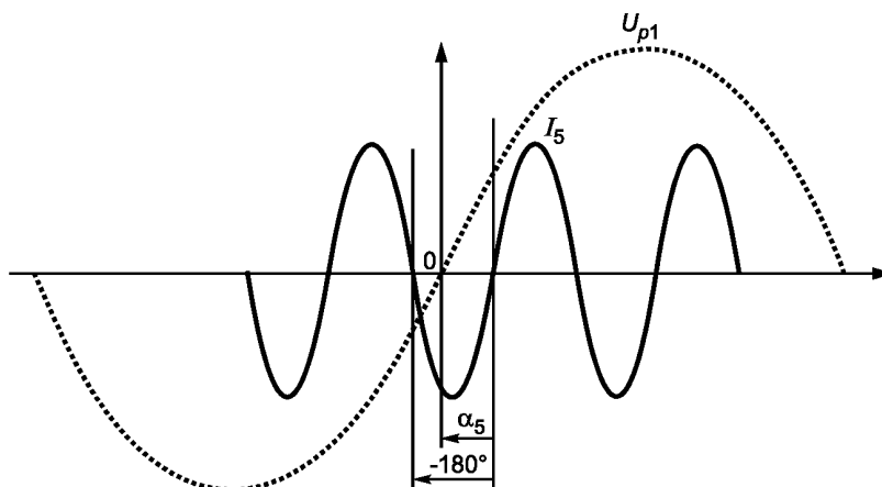
Рисунок 1 — Определение угла фазового сдвига гармонической составляющей тока 5-го порядка I_5 относительно основной составляющей фазного напряжения U_{p1} ( I_5 опережает U_{p1} , \alpha_5 > 0 )
