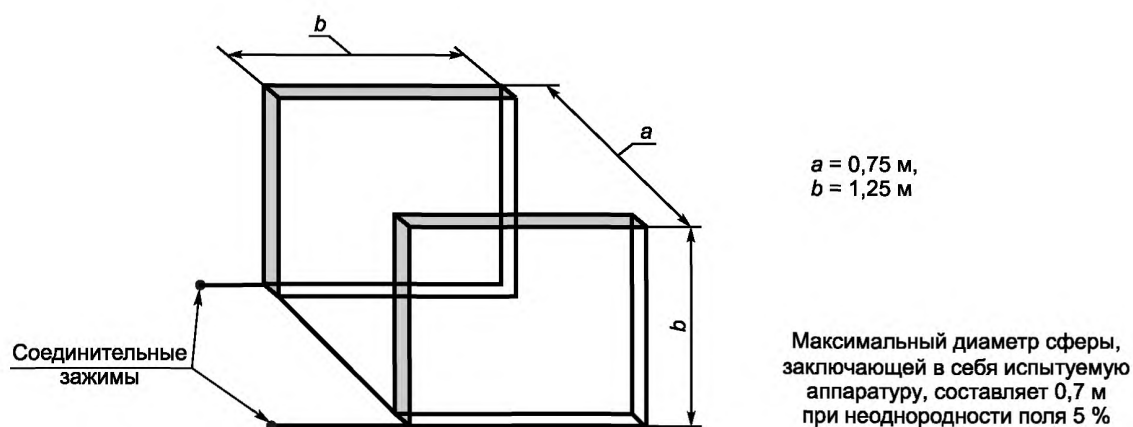
Рисунок А.1 — Конструкция катушек Гельмгольца для однородных полей
