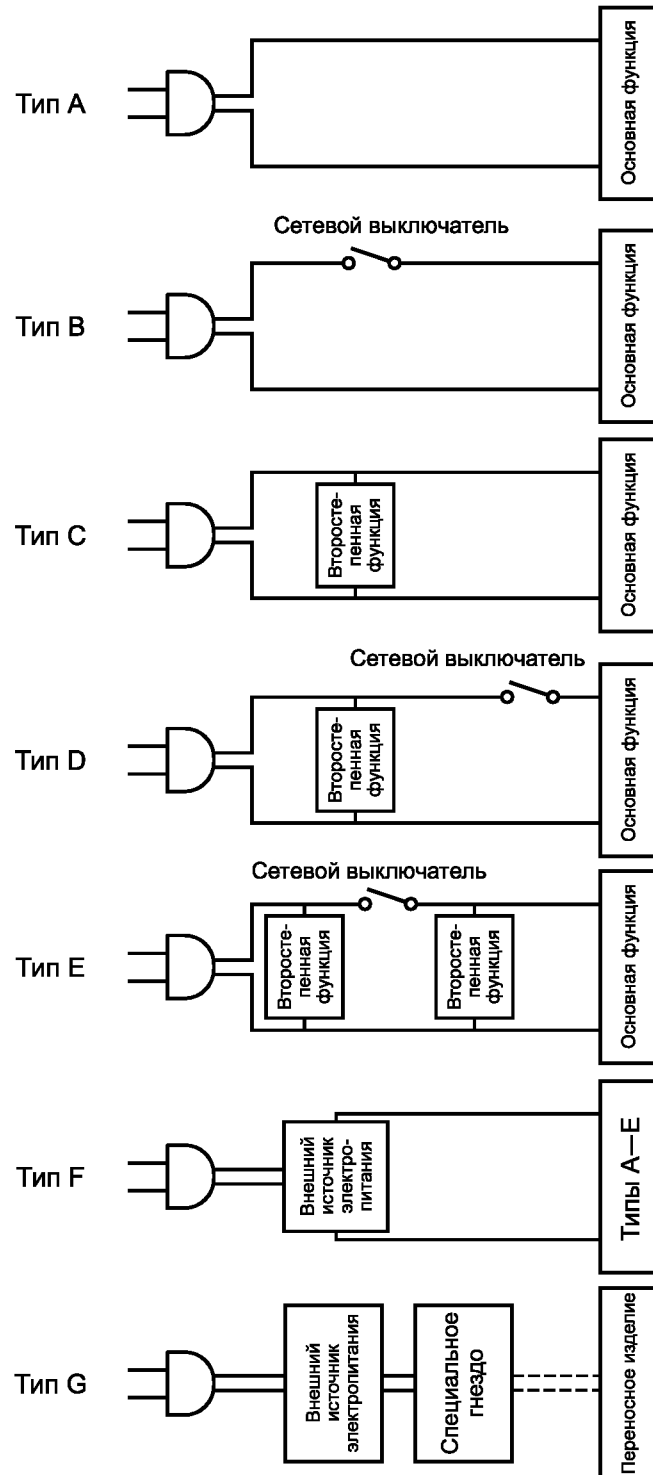
Рисунок А.1 — Принципиальные схемы типов приборов
