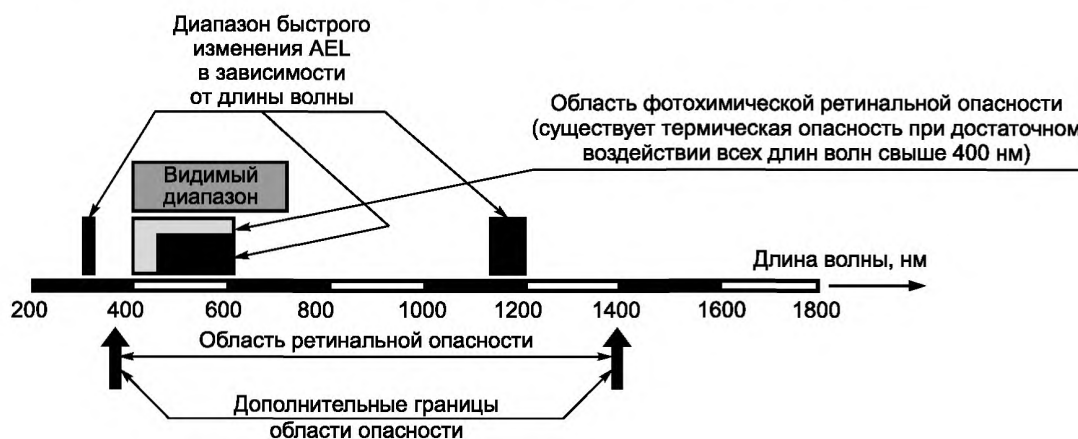
Рисунок 3 — Важные длины волн и диапазоны длин волн
