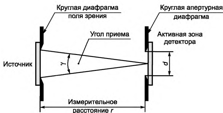
Рисунок 8b — Измерительная установка для доступного источника
