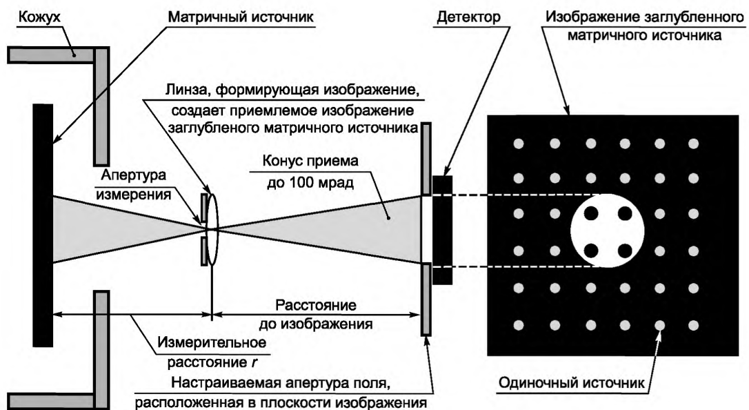
10b — Геометрия измерения для загнутого источника
