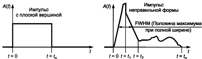
Рисунок 5 — Импульсы с плоской вершиной (плоские импульсы) и нерегулярные импульсы (импульсы неправильной формы)
