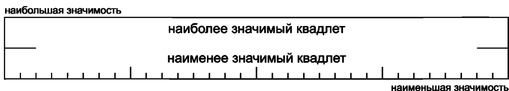
Рисунок 3 — Порядок следования квадлет в составе октлета
