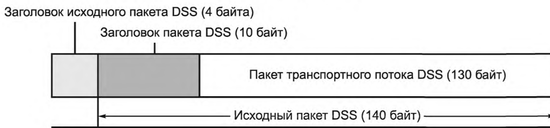
Рисунок 3 — Структура исходного пакета
