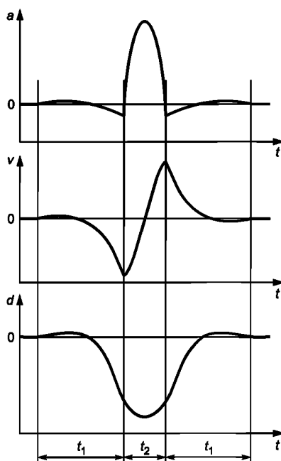
Рисунок А.2 — Сигналы ускорения, скорости и перемещения при воспроизведении ударного импульса полусинусоидальной формы с оптимизированными предупредными и послеударными участками
