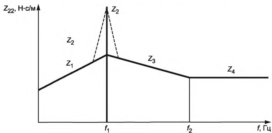
Рисунок А.4 — Типичная огибающая входных импедансов машины
