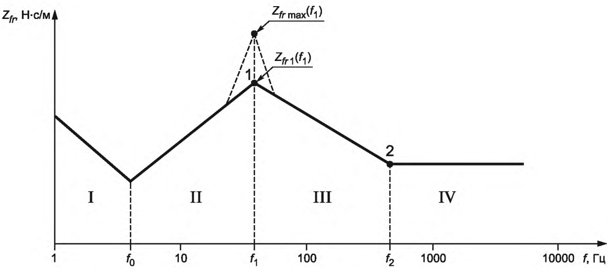
Рисунок А.6 — Типичная обходящая входных импедансов нагруженной рамы
