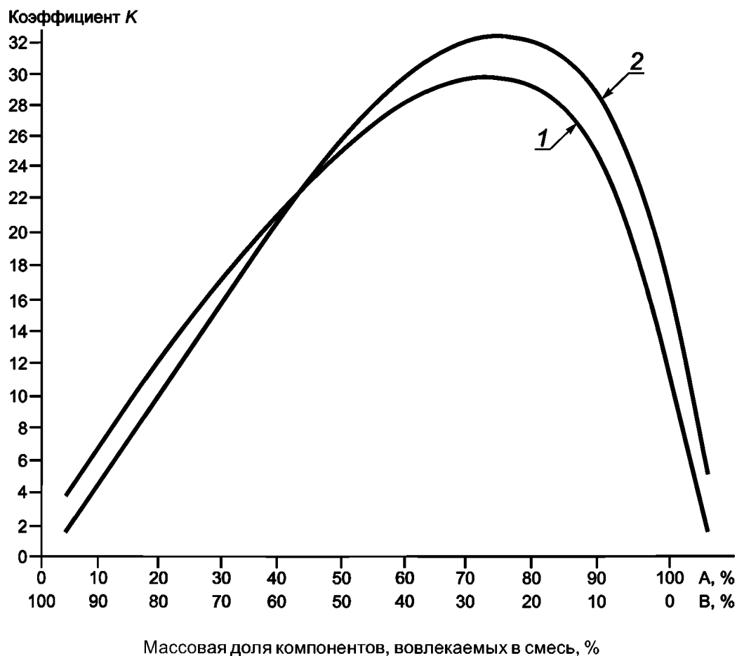
Рисунок 1 — Коэффициенты для вычисления значений вязкости (кривая 1) и температуры вспышки в закрытом тигле (кривая 2) смесей нефтепродуктов
