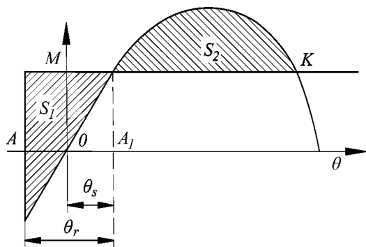
Рис. 1.2.2 Определение опрокидывающего момента плавучего крана в покоем состоянии по диаграмме статической остойчивости
