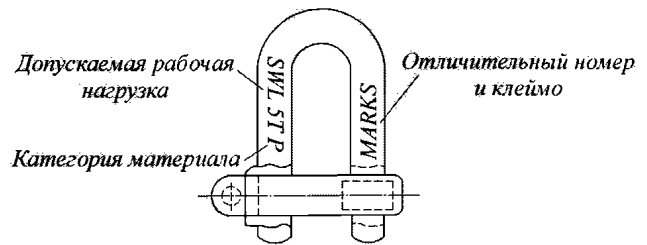
Рис. 11.2.1-3 Маркировка скобы
