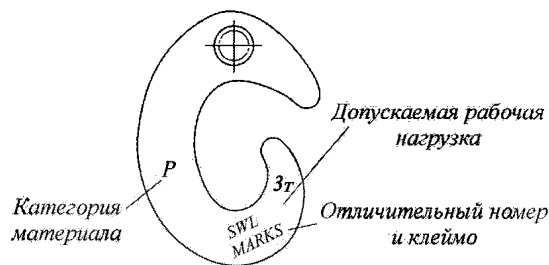
Рис. 11.2.1-1 Маркировка гака
