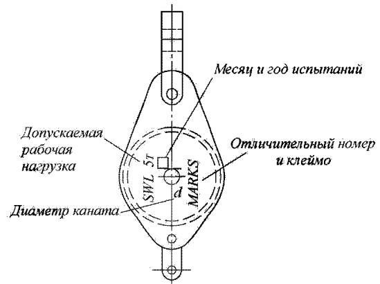
Рис. 11.2.1-5 Маркировка блока
