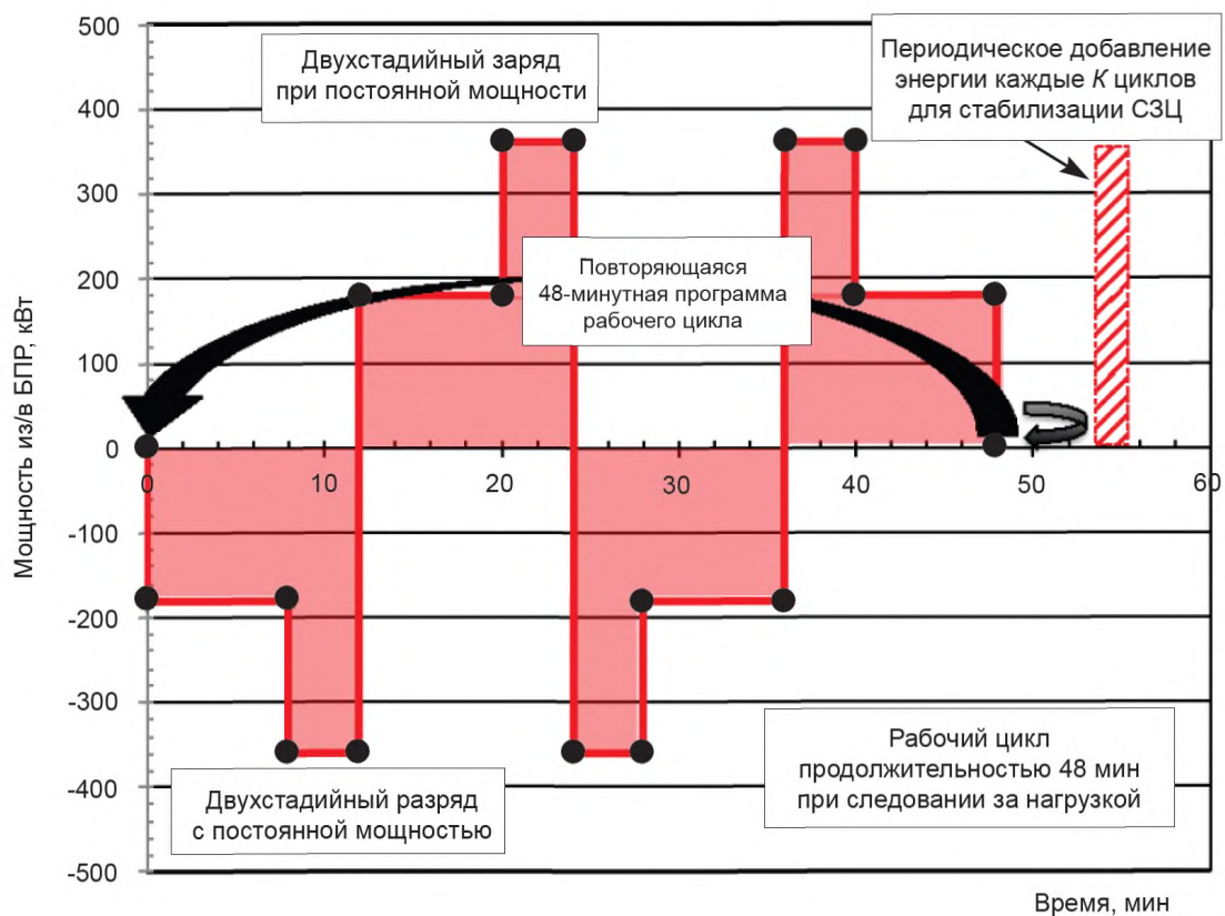
Рисунок 12 — Профиль программы работы в режиме следования за нагрузкой (см. 6.3) — профиль с
