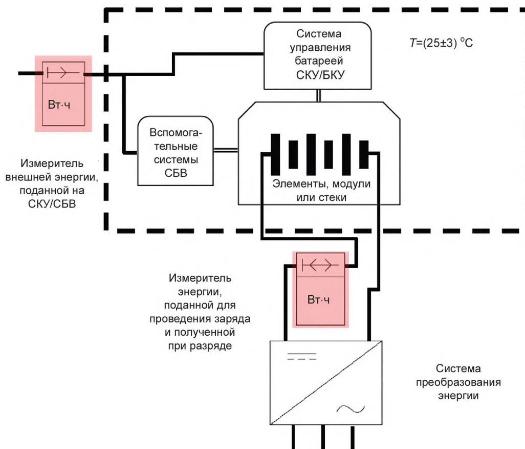
Рисунок 16 — Схематическое представление расположения двух точек измерения энергии (к вспомогательным системам и энергии к и от ОИБ) при определении \eta
