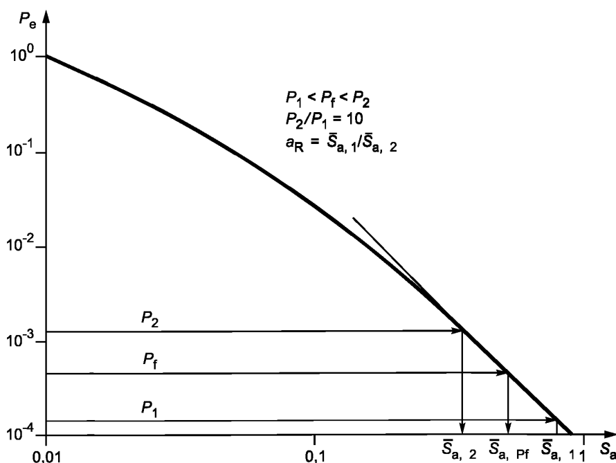
а) Определение наклона a_R кривой сейсмической опасности для T = T_{\text{dom}}
