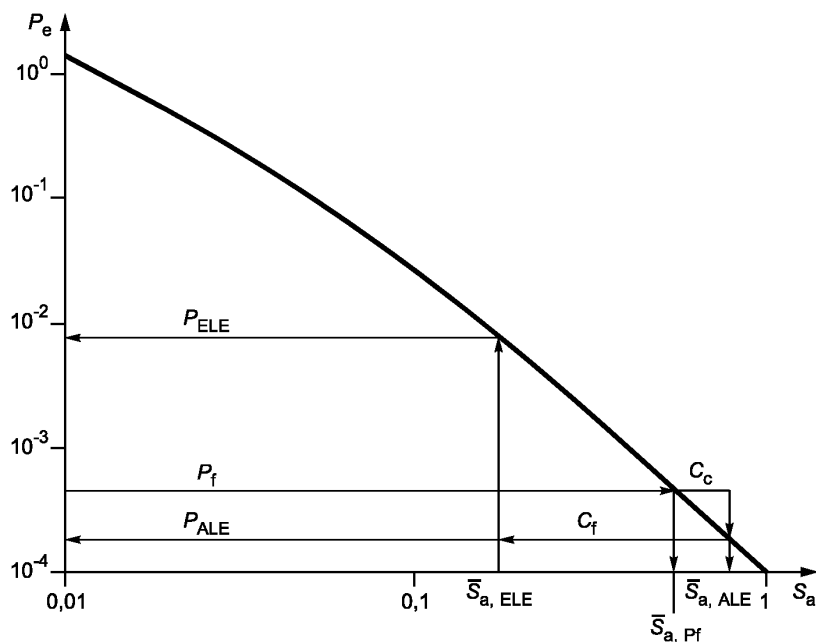
б) Определение спектральных ускорений и вероятностей для воздействий уровней МРЗ и ПЗ
