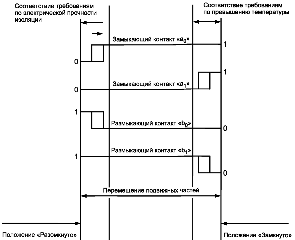
Рисунок А.1 — Взаимосвязь между вспомогательными контактами и устойчивыми положениями коммутационного компонента
