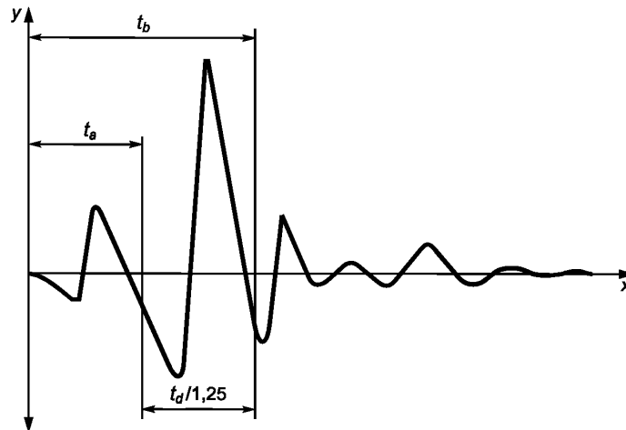
Рисунок 2 — Определение длительности импульса t_d
