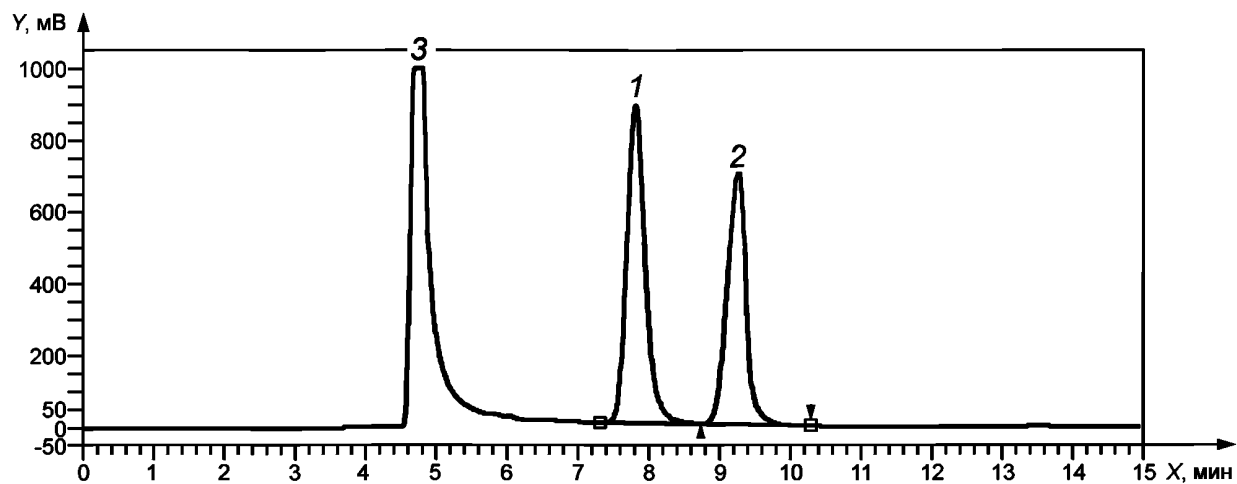
Рисунок В.2 — Пример хроматограммы
