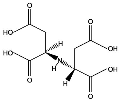
c) R,R-изомер
