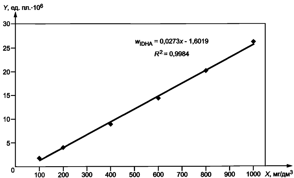
Рисунок В.3 — График градуировки
