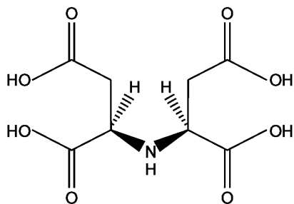
a) R,S-изомер
