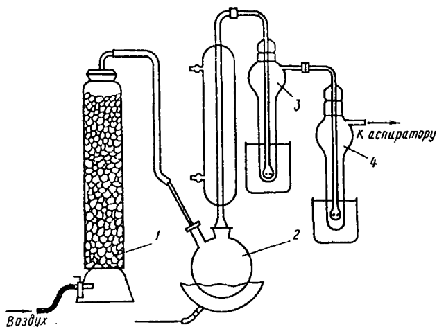
Рис. 1. Схема присоединения приборов: 1 — поглотительная колонка Фрезеннуса; 2 — колба с холодильником; 3 — поглотительный прибор, с 10%-ным раствором ацетата свинца; 4 — поглотительный прибор с 1,5%-ным раствором диэтиламина в спирте
