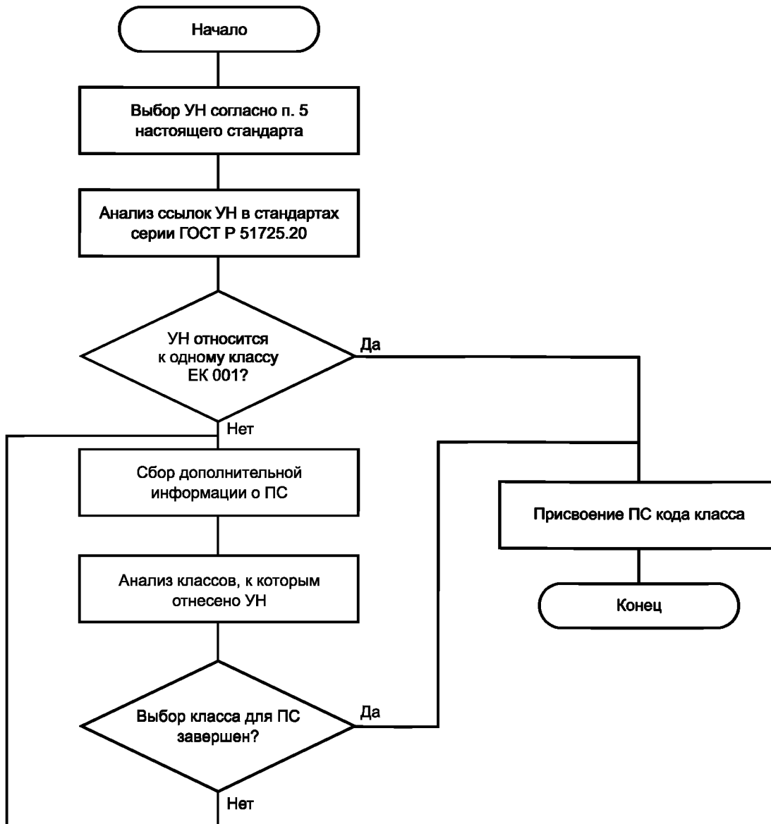
Рисунок 2 — Алгоритм классификации ПС
