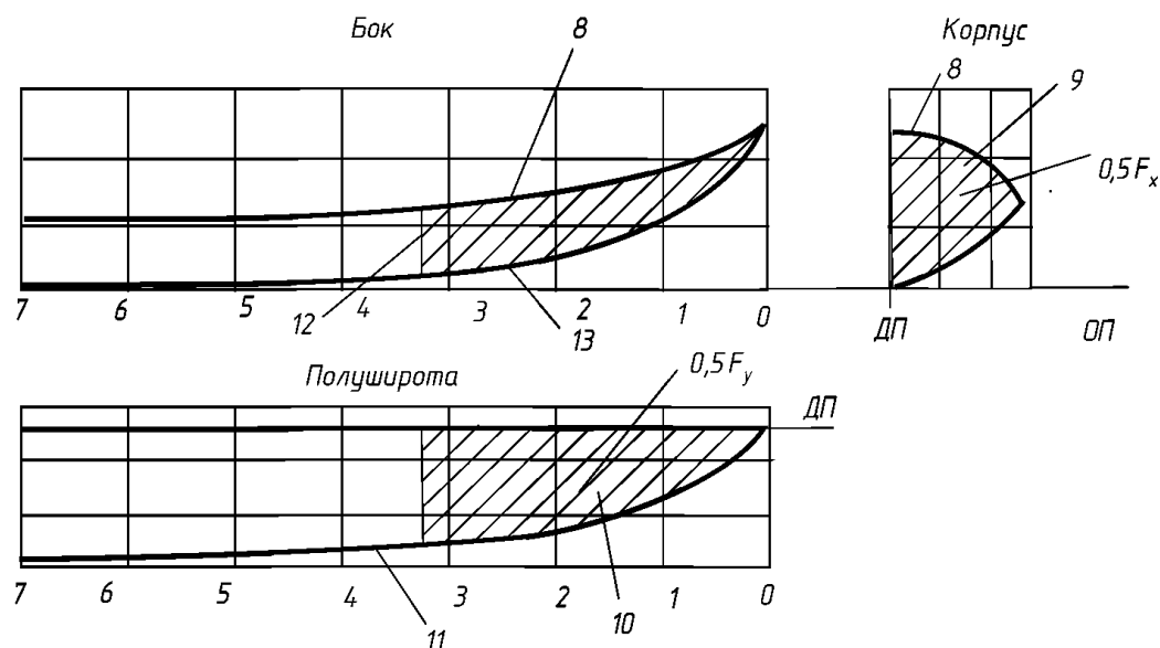
Рис. 2.3.8.2. Схема удара в носовую оконечность:
