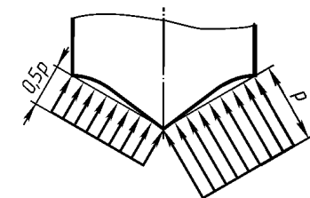
Рис. 2.7.8. Распределение давления в поперечном сечении экраноплана
