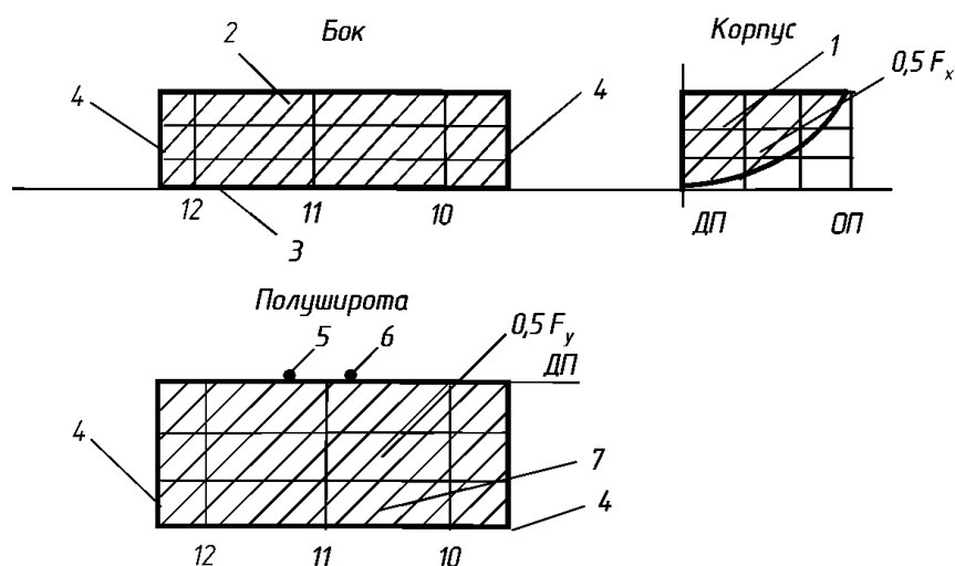
Рис. 2.3.9.2. Схема удара в район центра масс:
