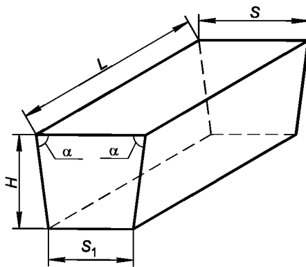
Рисунок 1 — Ребровый двусторонний клин
