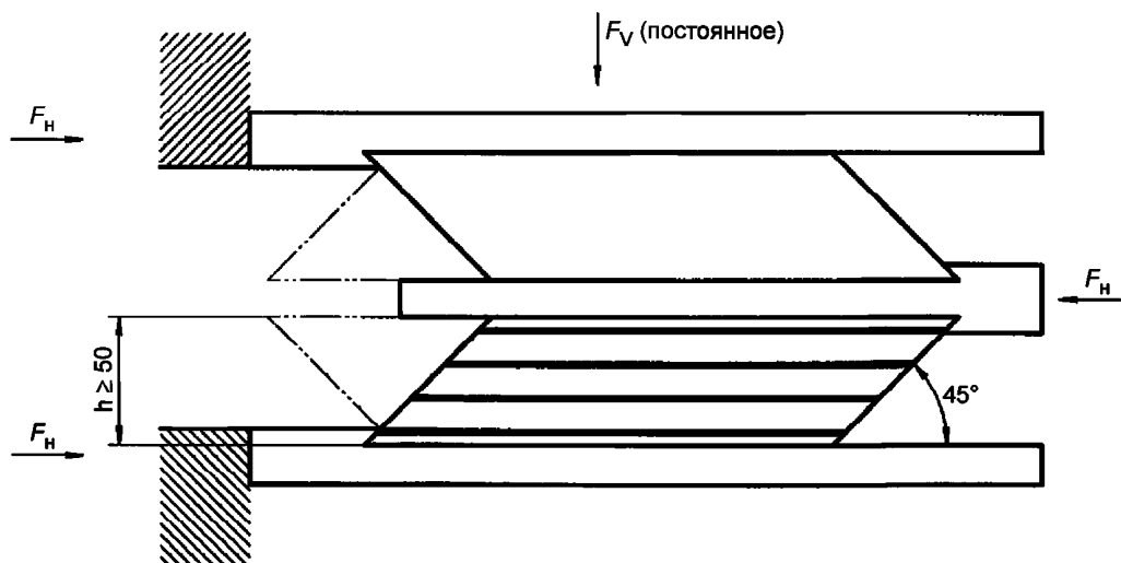
Рисунок А.1 — Образцы для испытания на «сдвиг—разрушение»
