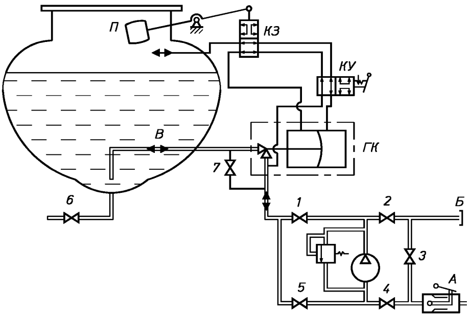
1—6 — задвижки; 7 — вентиль; А — напорно-всасывающий патрубок; Б — напорный патрубок; В — трубопровод для наполнения и опорожнения; ГК — гидроклапан; П — поплавок; КЗ — кран золотниковый; КУ — кран управления
